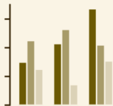
Grouped Bars
